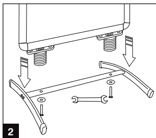
2 Fixar a moldura na base (chave incluída)
